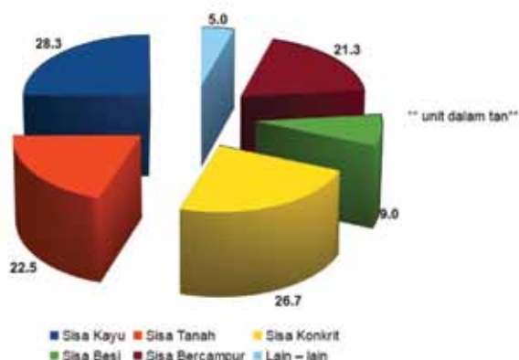
Rajah 1: Komposisi sisa pepejal pembinaan yang dihasilkan di tapak bina semasa kajian
